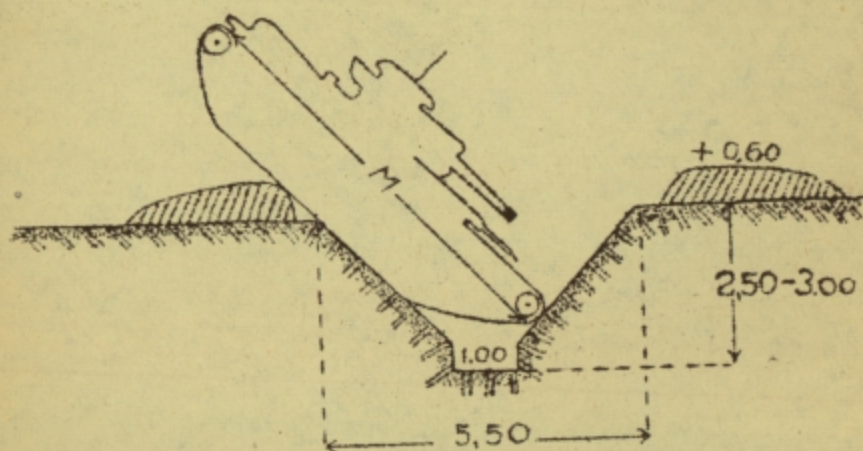
ΣΧ. 5 ΑΝΤΙΑΡΜΑΤΙΚΗ ΤΑΦΡΟΣ ΜΕ ΚΛΙΣΗ 45° (ΔΥΟ ΚΑΤΕΥΘΥΝΣΕΩΝ)
