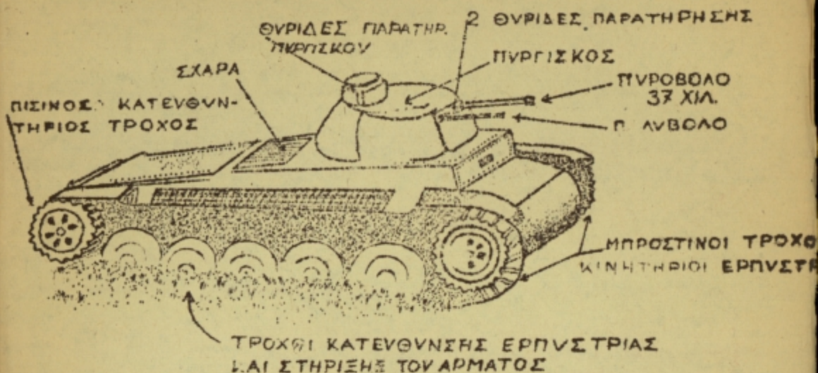
ΣΧ.1. ΣΤΟΙΧΕΙΩΔΗ ΜΕΡΗ ΤΟΥ ΑΡΜΑΤΟΣ ΜΑΧΗΣ
