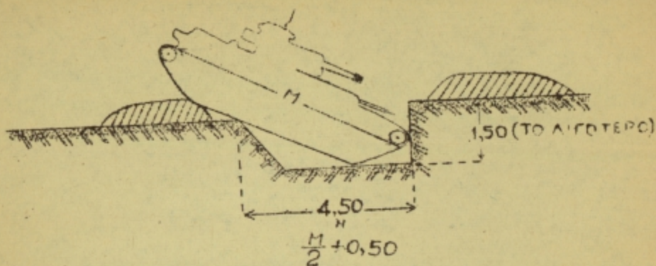
ΣΧ. 4 ΑΝΤΙΑΡΜΑΤΙΚΗ ΤΑΦΡΟΣ ΜΙΑΣ ΚΑΤΕΥΘΥΝΣΗΣ
